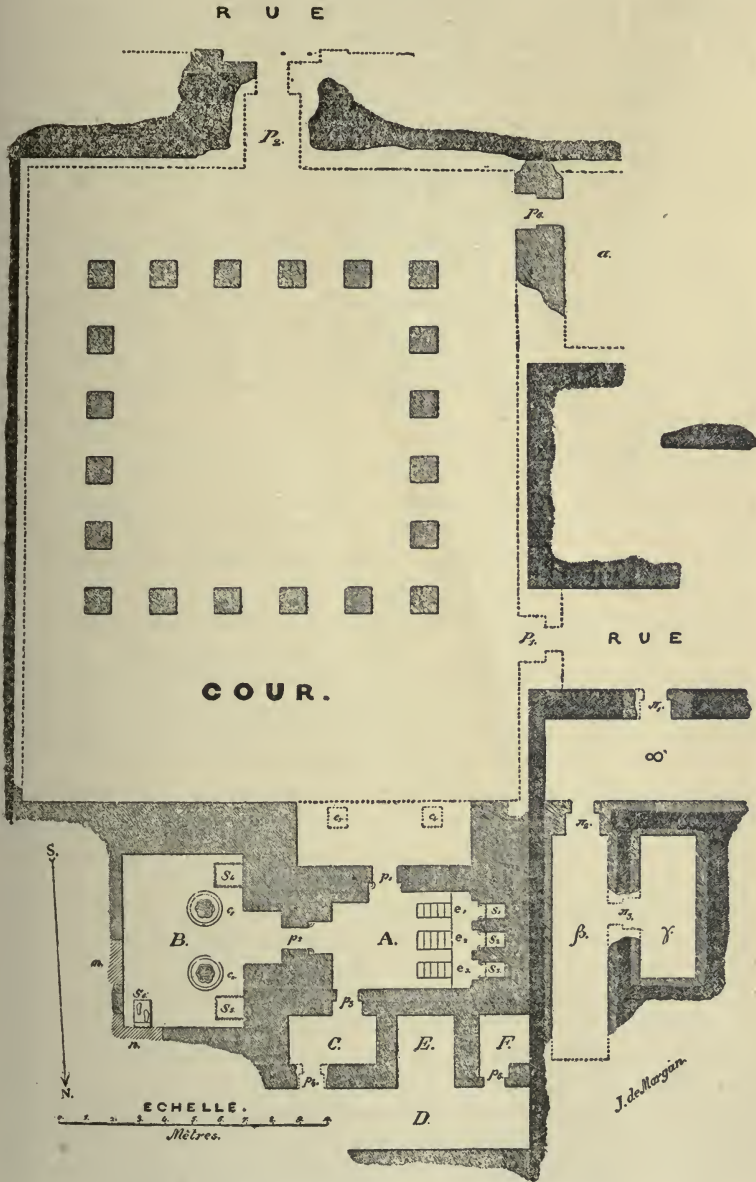
FIG. 2.—PLAN OF THE MASTABA OF PTAH-SHEPSÊS.
